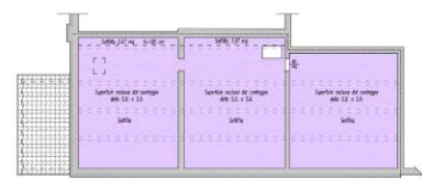
piano sottotetto
